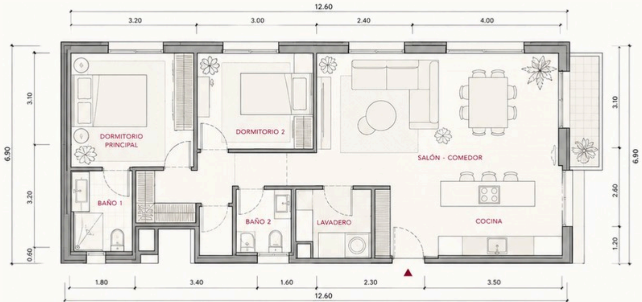
PLANO ACOTADO Y DISTRIBUCIÓN
